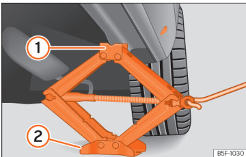
Afb. 229 Langsligger: plaatsing van de wagenkrik.
