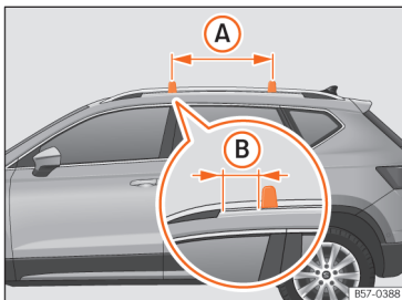
Afb. 182 Bevestigingspunten voor de reling van het dakdragersysteem
