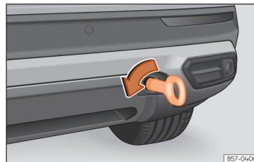
Afb. 200 Aan de rechterzijde van de achterbumper: vastgeschroefd sleepoog.
