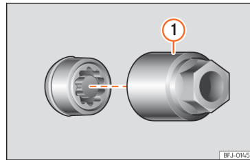
Afb. 225 Wielbout met diefstalbeveiliging, voorzien van dop en adapter.
