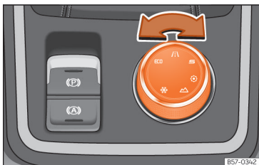
Afb. 105 Middenconsole: draaiknop (Driving Experience button).
