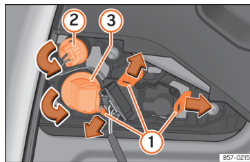
Afb. 206 Fitting uitbouwen.
