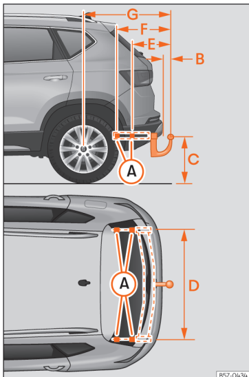
Afb. 187 Maten en bevestigingspunten voor het achteraf inbouwen van een trekhaak.
