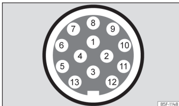
Afb. 183 Schematische weergave: toewijzing van de pinnen van het stopcontact voor de aanhangwag en.
