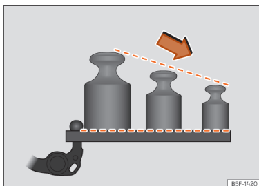
Afb. 185 Aanbevolen verdeling van het gewicht in het draagsysteem achteraan.
